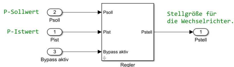
Abbildung 13: Wirkleistungsregler
