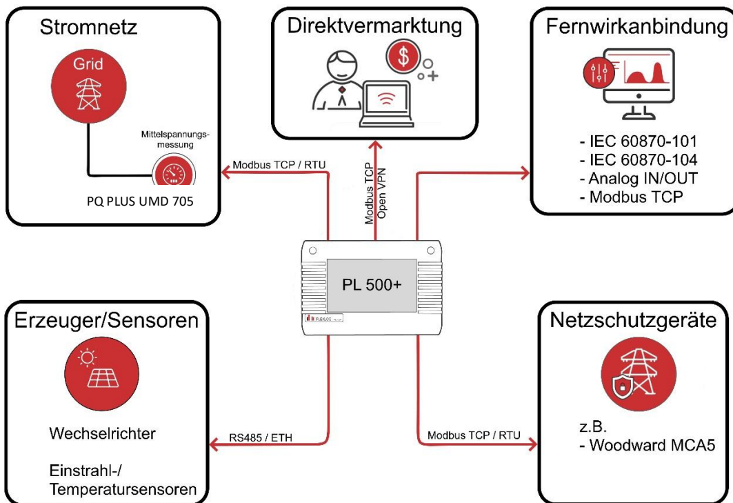
Abbildung Blockschaubild EZA-Regler PL500+
