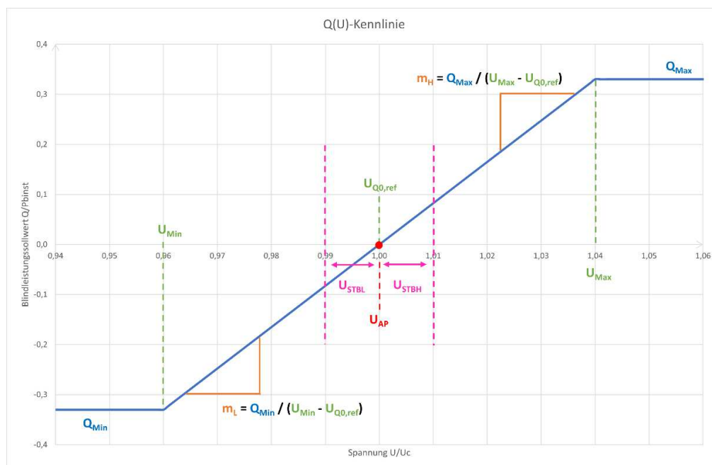
Abbildung 5: Kennlinie Verfahren a)
