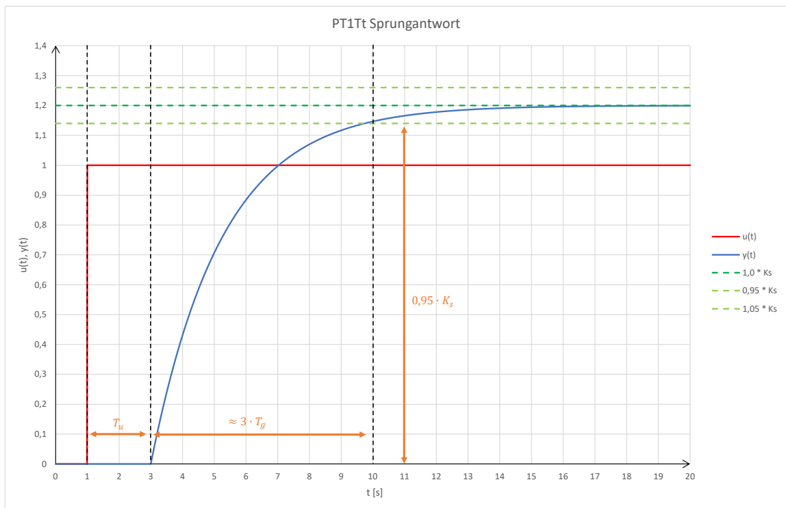
Abbildung 19: PT1Tt - Sprungantwort
