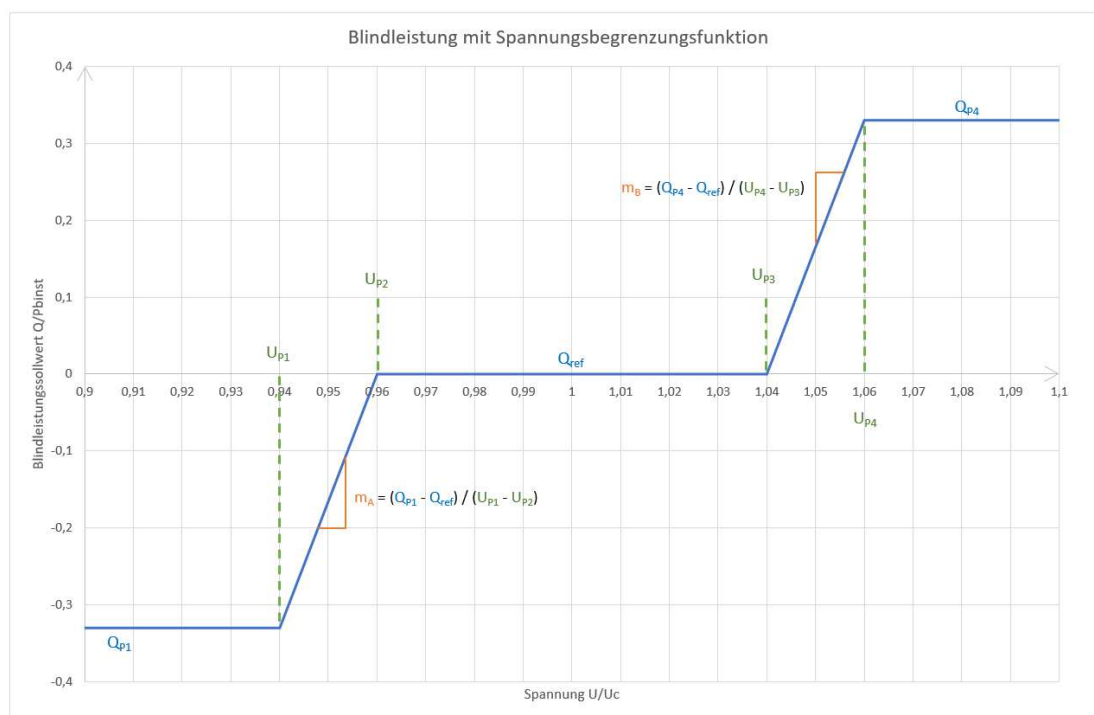
Abbildung 10: Kennlinie Verfahren c)
