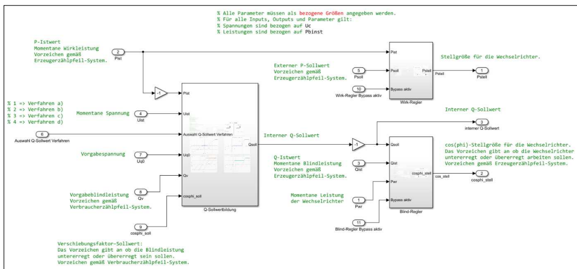
Abbildung 2: Die drei internen Blöcke des EZA-Reglers
