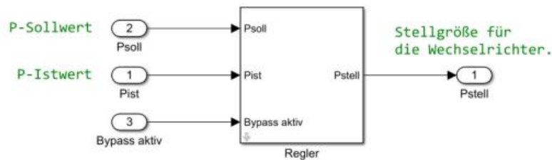
Abbildung 13: Wirkleistungsregler
