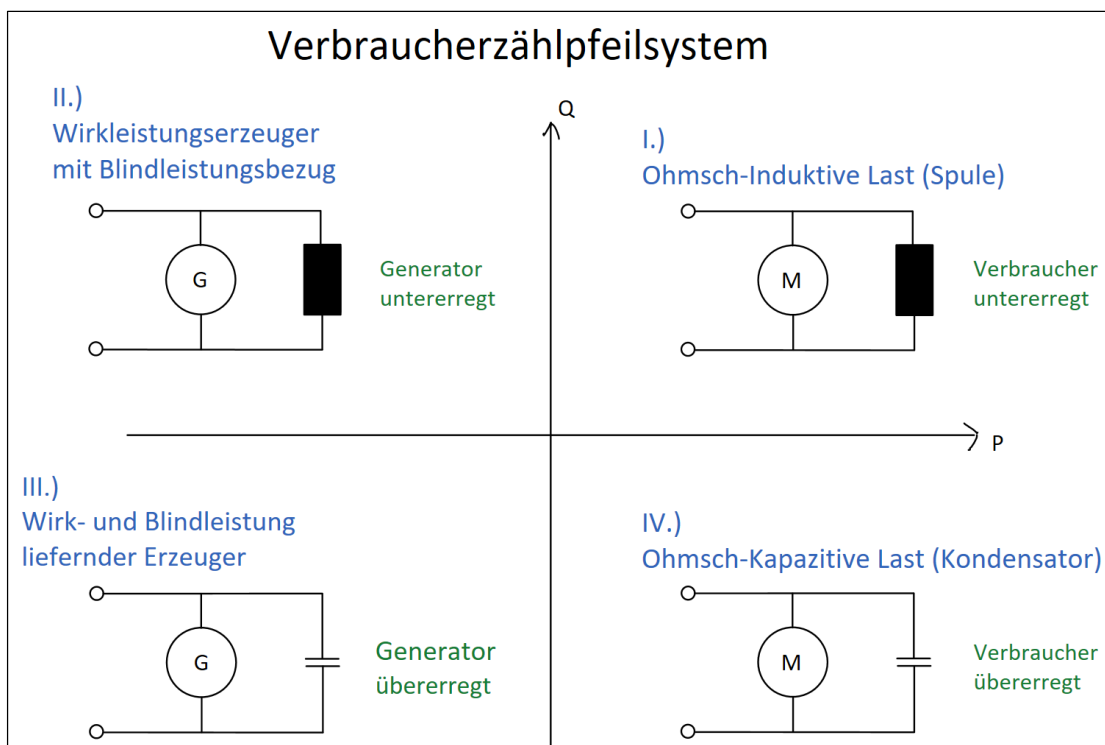
Abbildung 21: Verbraucherzählfeilsystem
