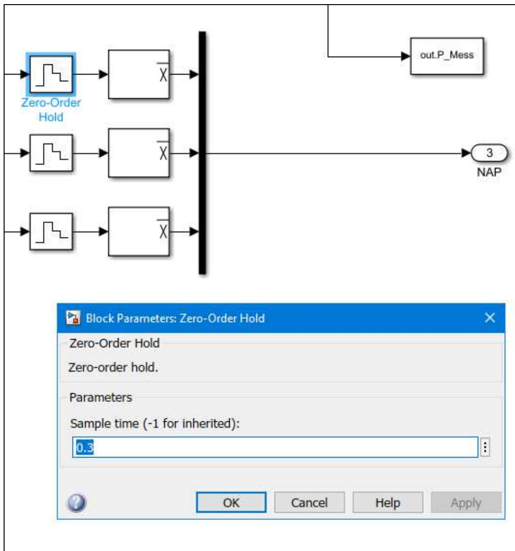
Abbildung 27: Abtastzeit des Netzanalysegeräts
