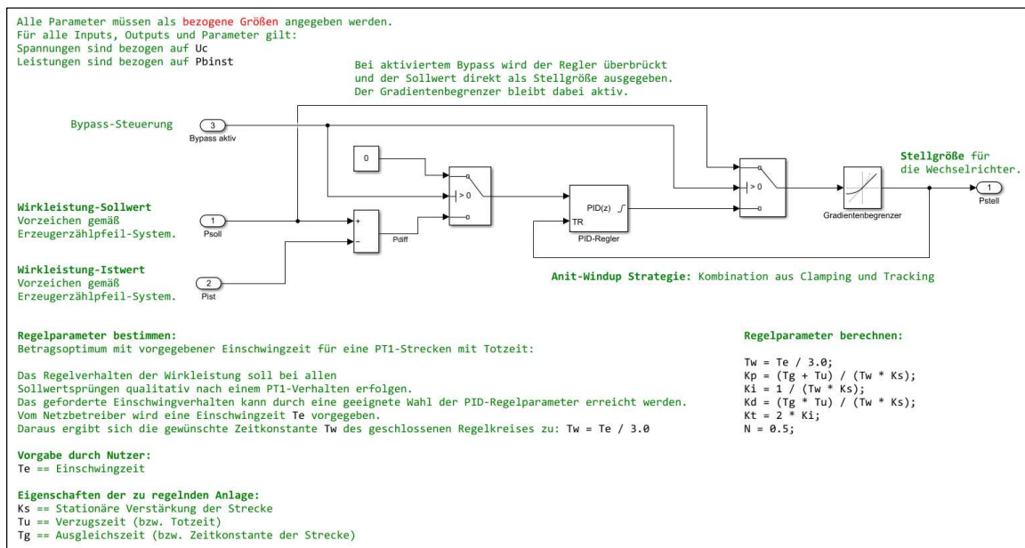
Abbildung 14: Wirkleistungsregelalgorithmus
