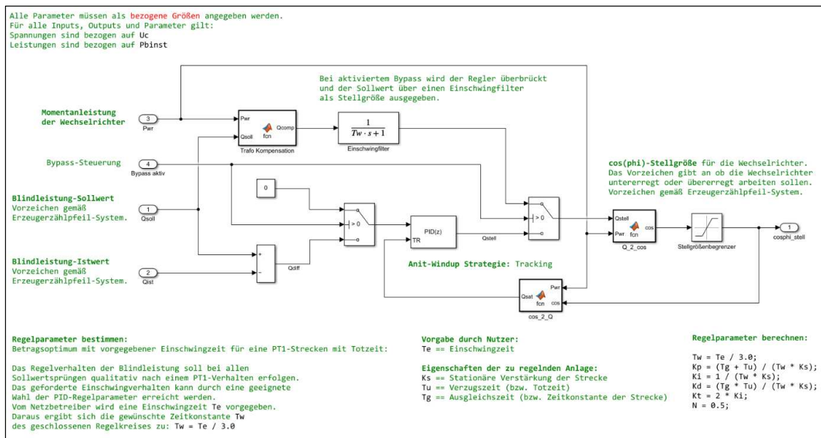
Abbildung 17: Blindleistungsregelalgorithmus
