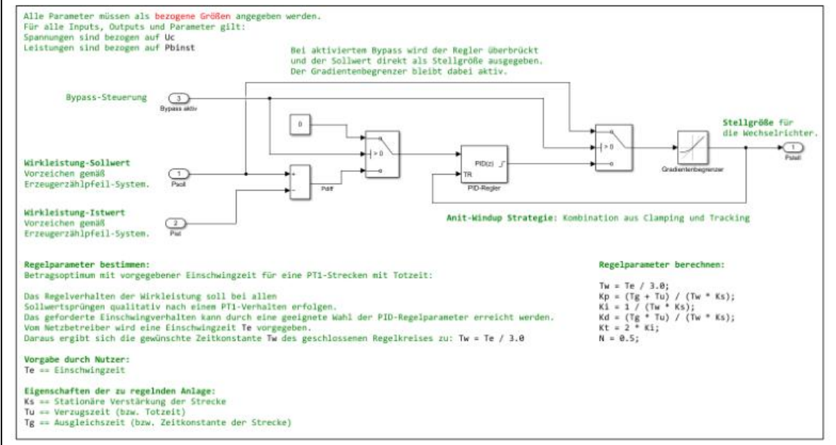
Abbildung 3.1.4 Umsetzung des Wirkleistungsmanagement (Quelle: Anhang 1, Modellbeschreibung)
