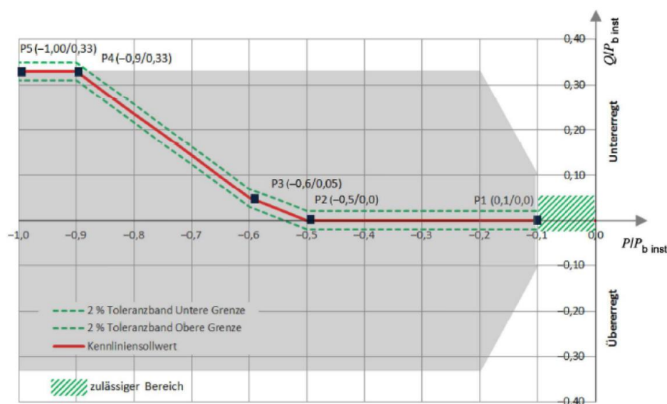
Abbildung 8: Kennlinie Verfahren b)
