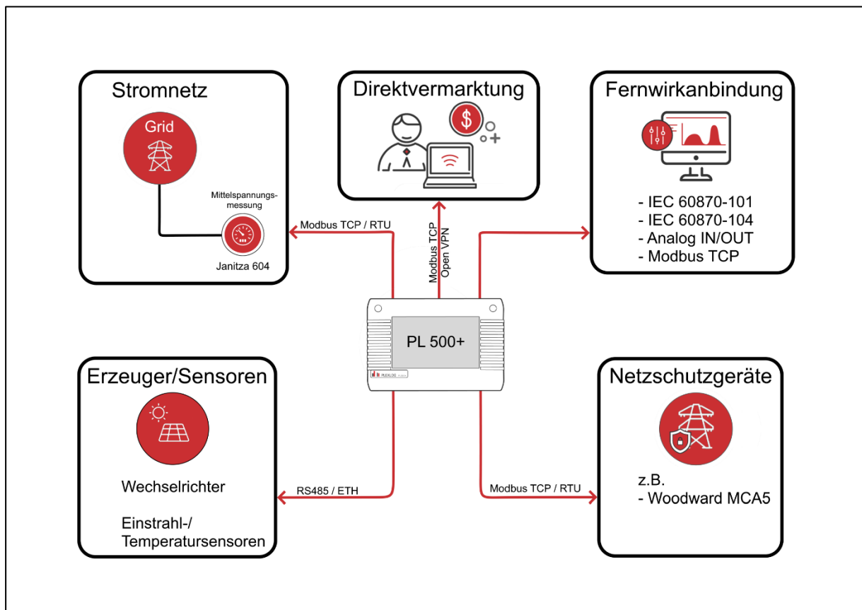
Abbildung 3.1.5 Schematischer Aufbau der Einbindung des EZA-Reglers (Quelle: Anhang 1, Herstellererklärung)
