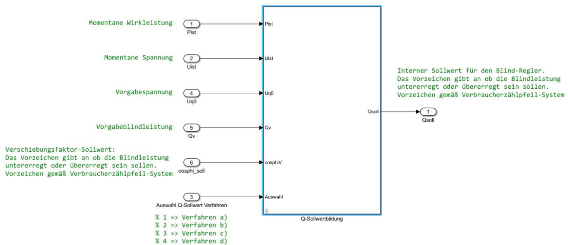
Abbildung 3: Der Block Q-Sollwertbildung
