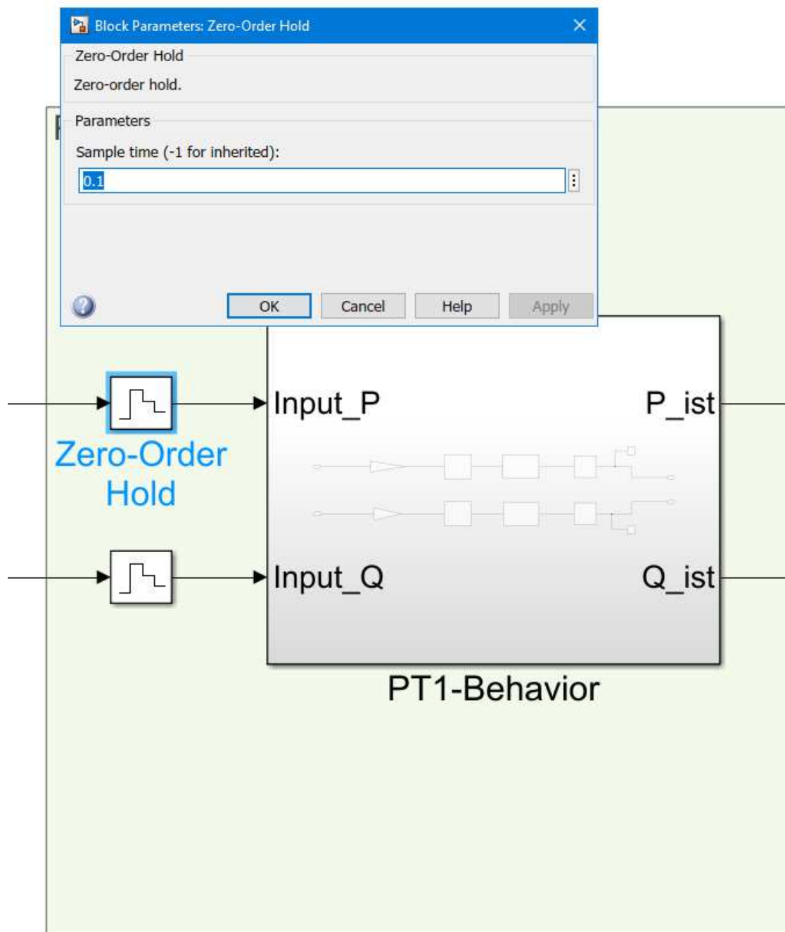
Abbildung 26: Sende-Intervall Regler
