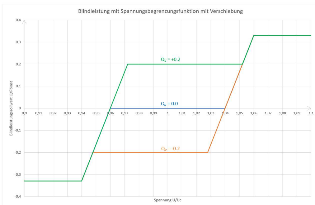
Abbildung 12: Kennlinienverschiebung Verfahren c)
