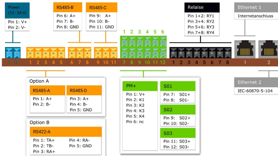
Abbildung 3.1.2 Anschlussbelegung der Komponente (Quelle: Kapitel 2.2)
