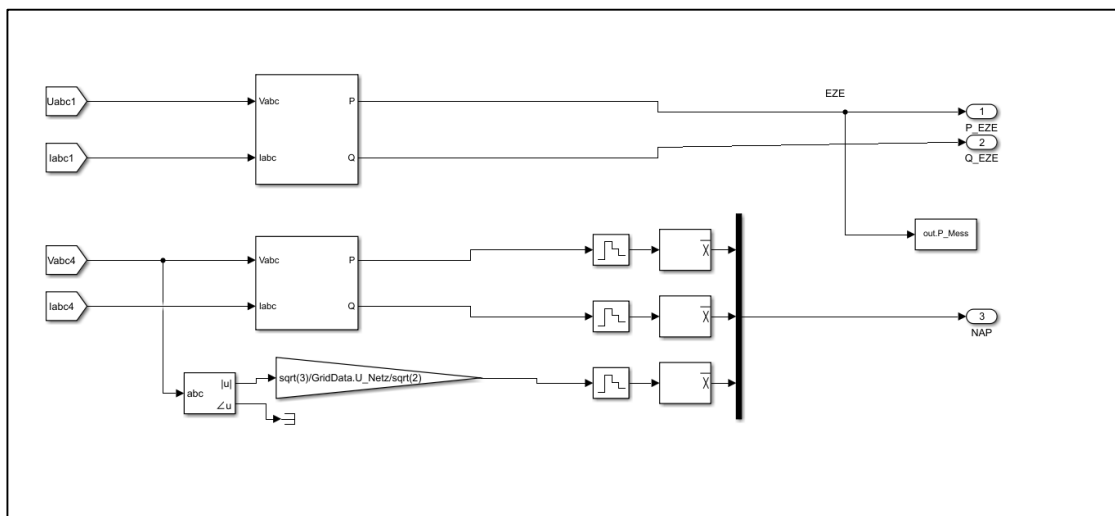
Abbildung 25: Netzanalysegerät
