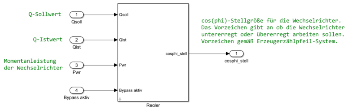
Abbildung 16: Blindleistungsregler
