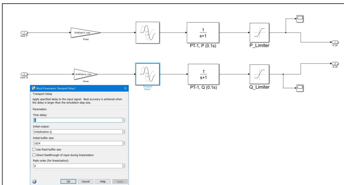
Abbildung 29: Nachbildung Zeitverhalten EZE und Umrechnung in Absolutgrößen
