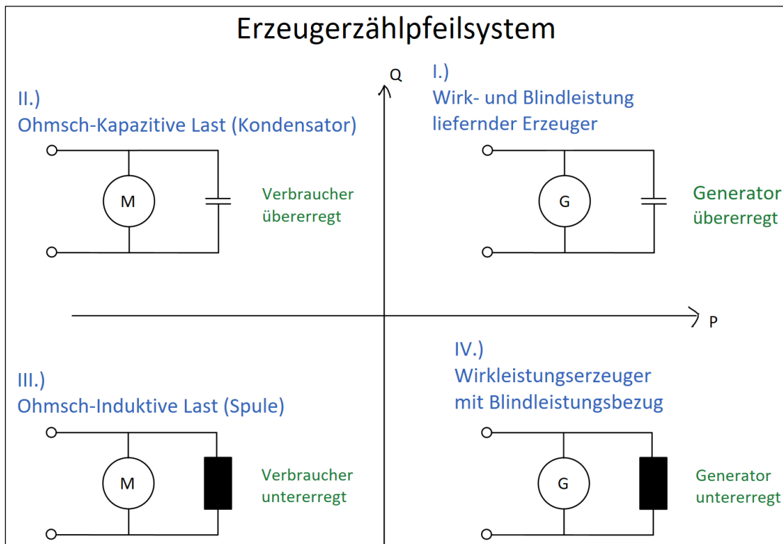
Abbildung 20: Erzeugerzählfeilsystem
